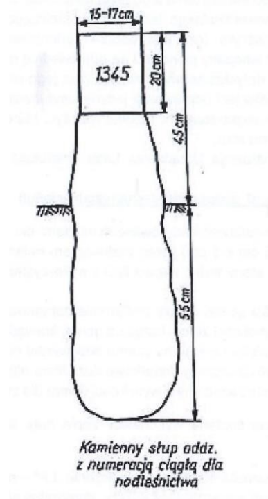
Rysunek 1. Parametry słupka kamiennego wraz z oznaczeniem słupka oddziałowego.
